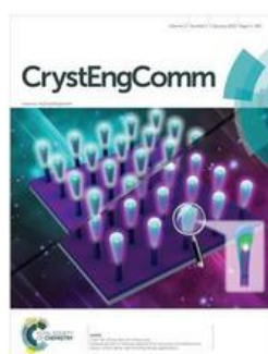
CrystEngComm
